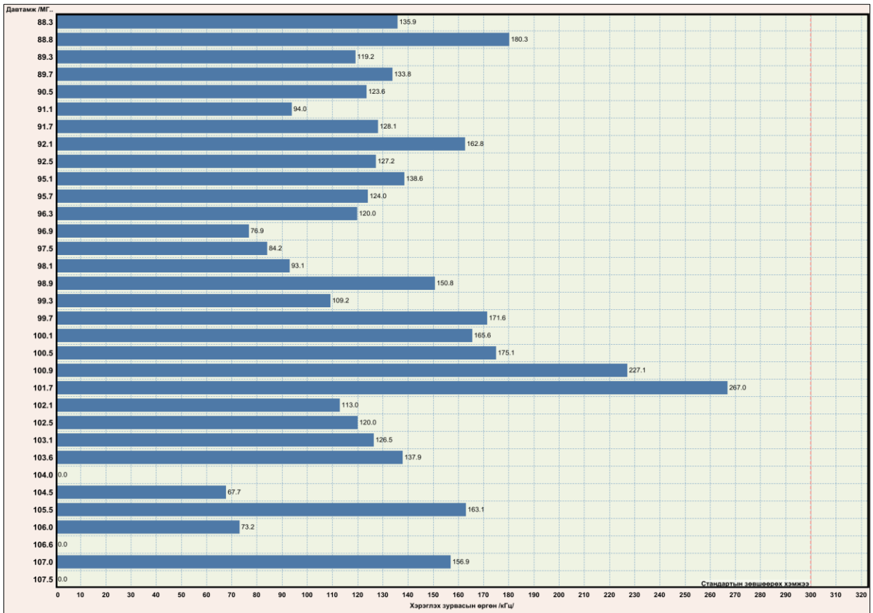
Зураг 4. Хэрэглэх зурвасын өргөний хэмжилтийн үр дүн.
