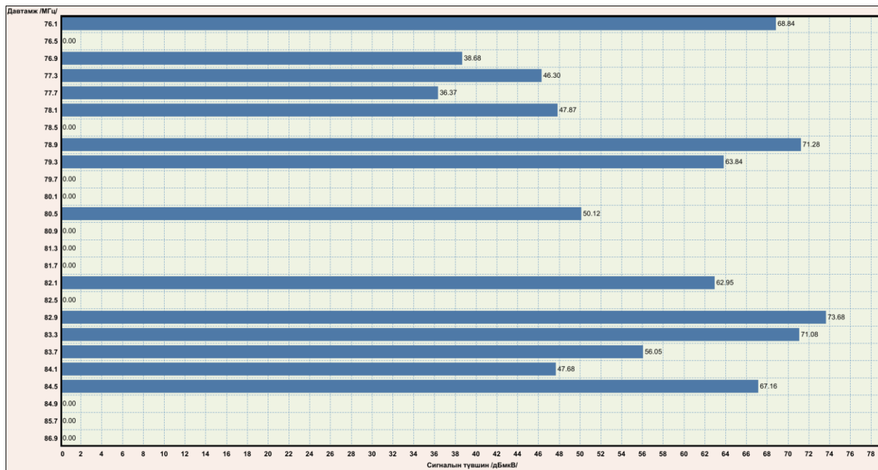
Зураг 8. Радио давтамжийн 75-88 МГц-ийн зурваст хэмжигдсэн дохионы түвшин.
