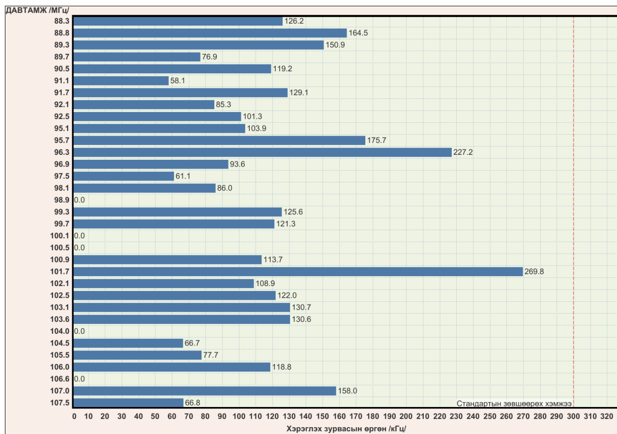
Зураг 5. Хэрэглэх зурвасын өргөний хэмжилтийн үр дүн
