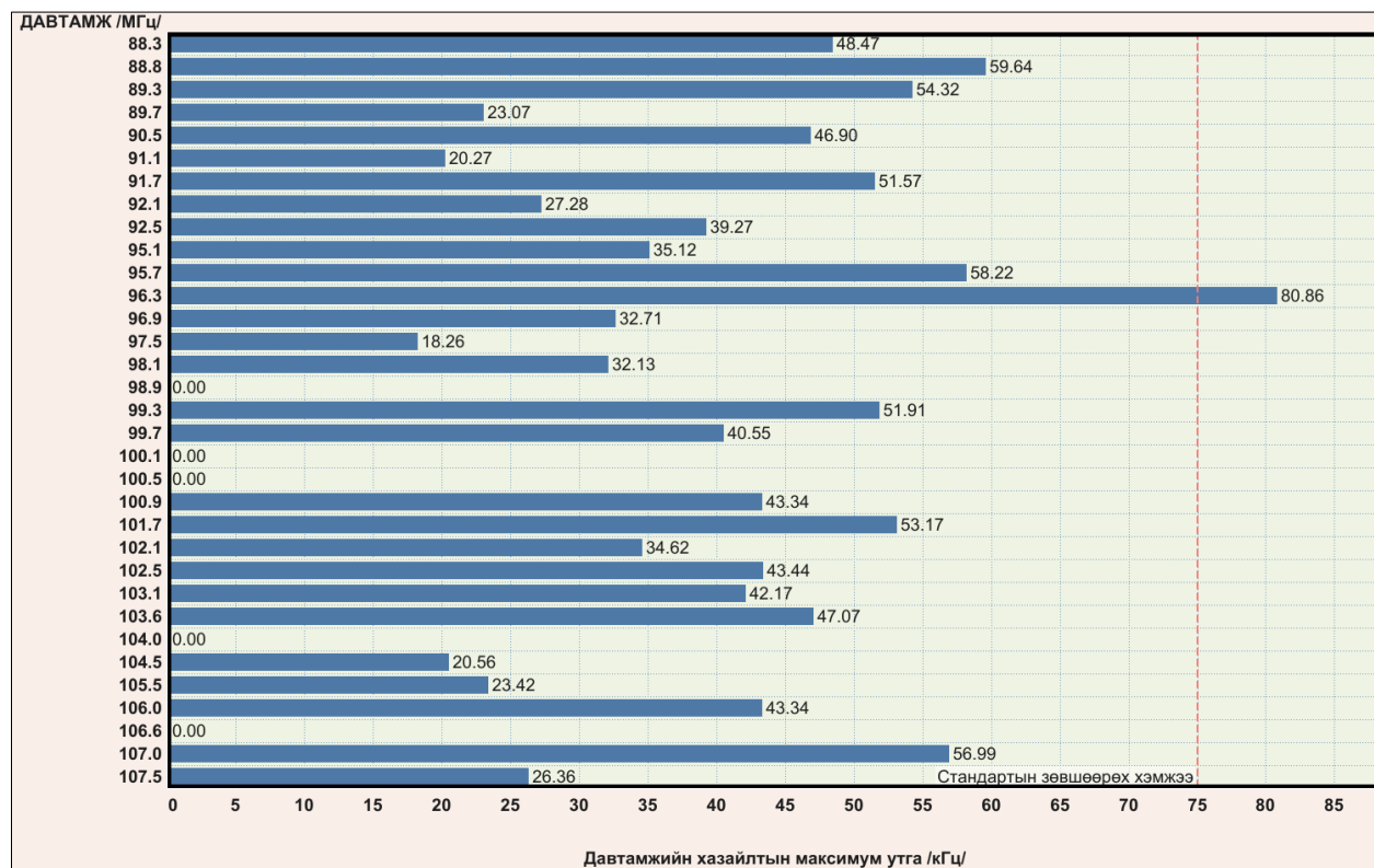
Зураг 6. Давтамжийн хазайлтын максимум утгын хэмжилтийн үр дүн
