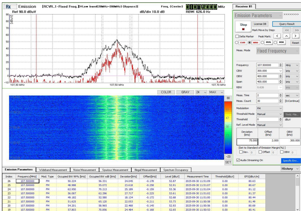
Зураг 3. FM радио станцад хэмжилт хийж байгаа нь
