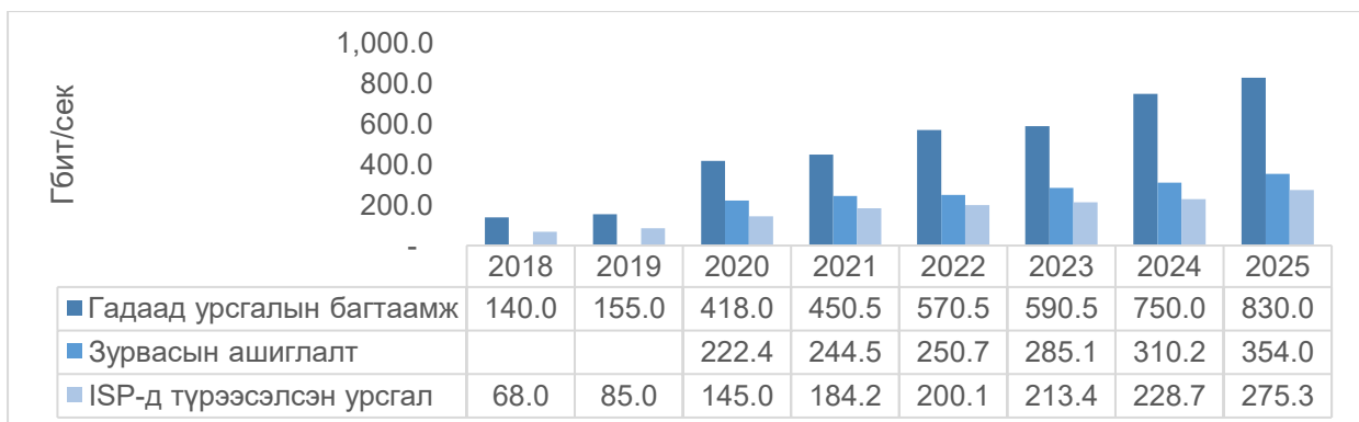
Зураг 8. Интернэтийн бөөний үйлчилгээ эрхлэгчдийн нийт урсгалын багтаамж: Гбит/сек
