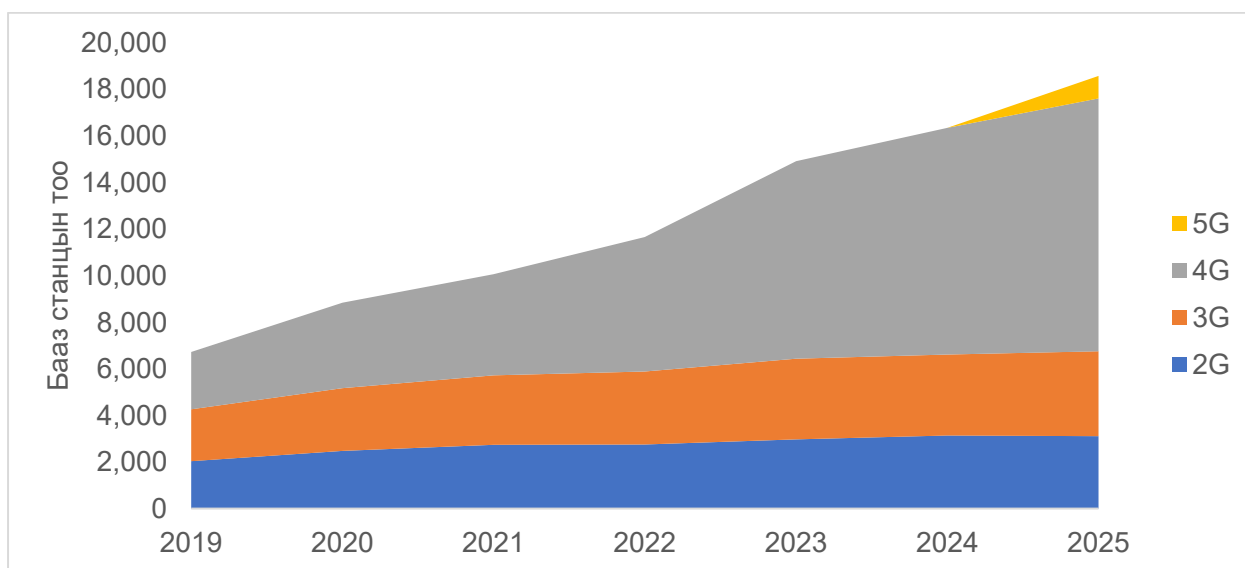
Зураг 14. Үүрэн холбооны бааз станцын тоо, технологийн төрлөөр
