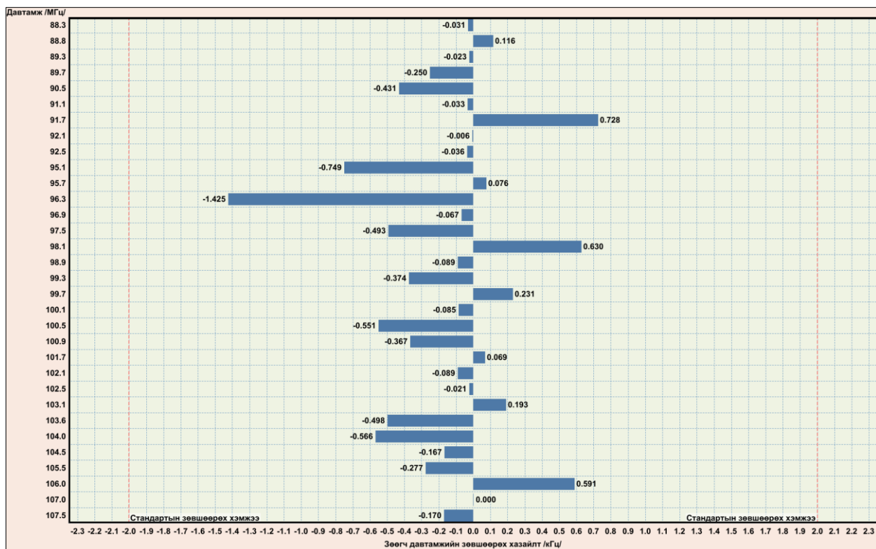
Зураг 5. Зөөгч давтамжийн зөвшөөрөх хазайлтын хэмжилтийн үр дүн
