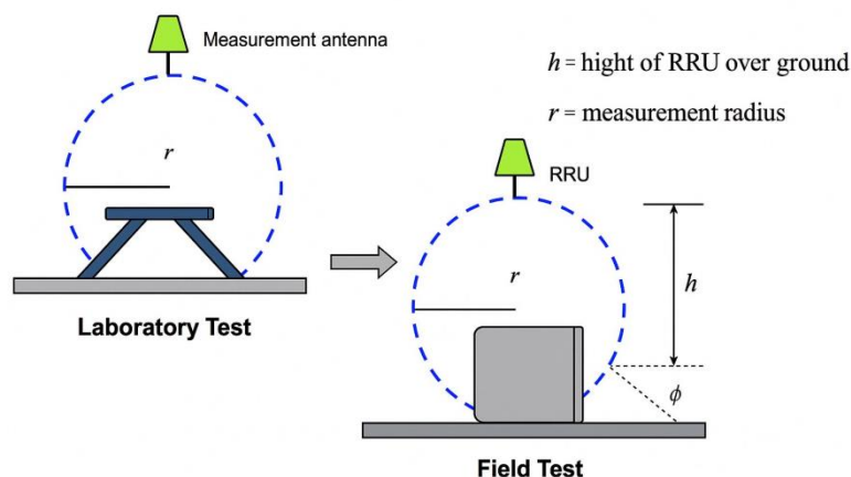
6.5.2-р зураг - Лабораторийн болон гадна талбайд цацаргалтын бүх хэмжилтийг (TE, UE, OE, UE-TP) хийх
