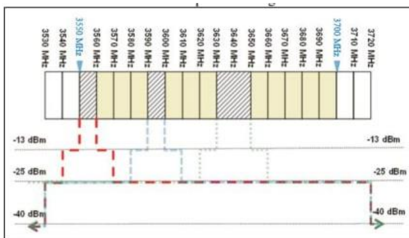
Х.3.11.2-р зураг - Олгогдсон сувгуудын цацаргалтын хязгаар
