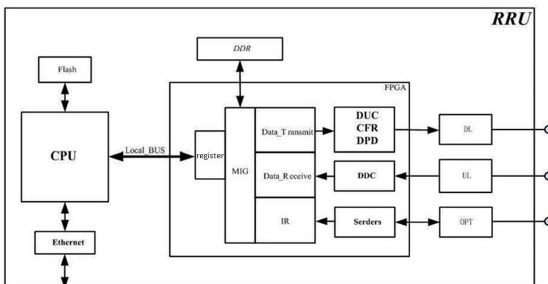
Х.4.1-р зураг - RRU хэмжилтийн системийн бүдүүвч
