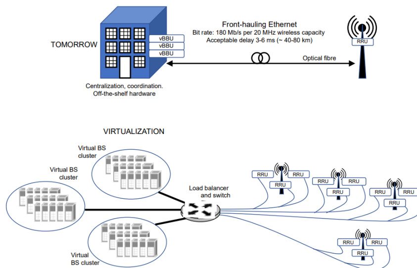
Х.1.3-р зураг - V-RAN ба холболтын интерфейсын бүтэц
