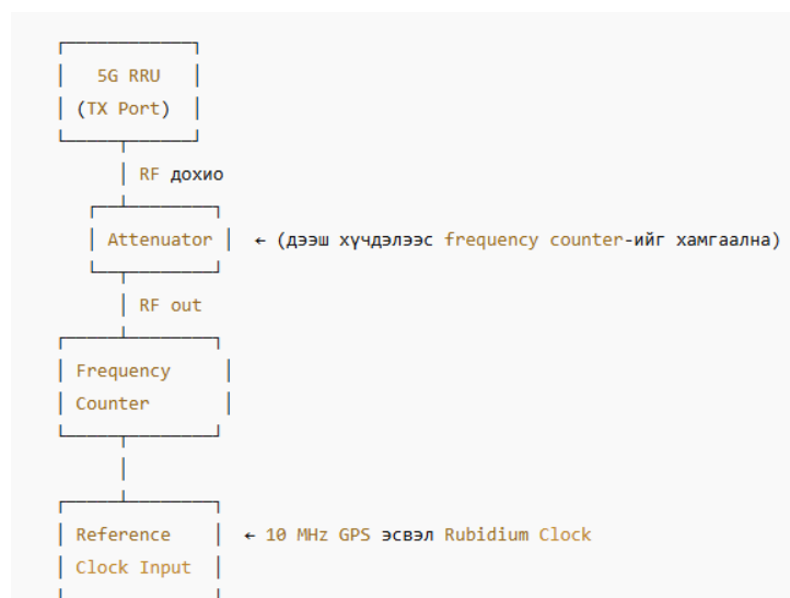
Зураг 7.9.1 5G RRU → Frequency Counter ашиглан давтамжийн алдааг хэмжих ерөнхий холболтын схем
