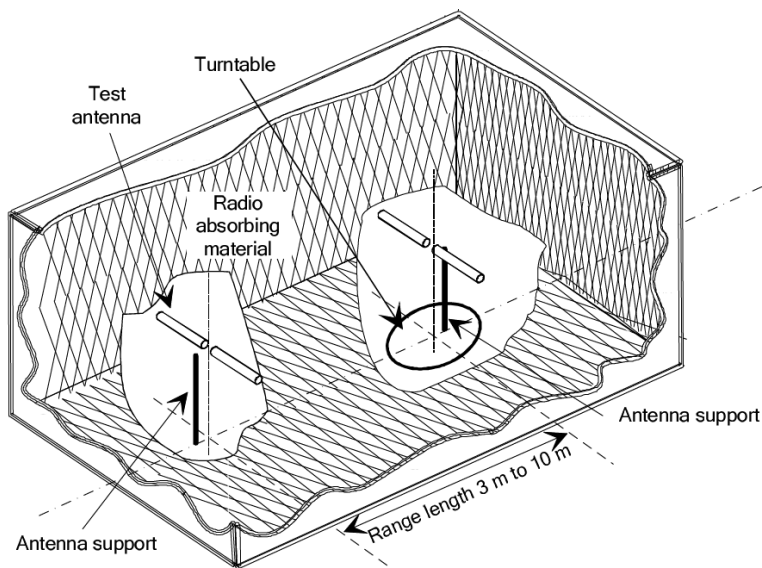
Х.3.1А-р зураг - Ердийн цуурайгүй чембер
