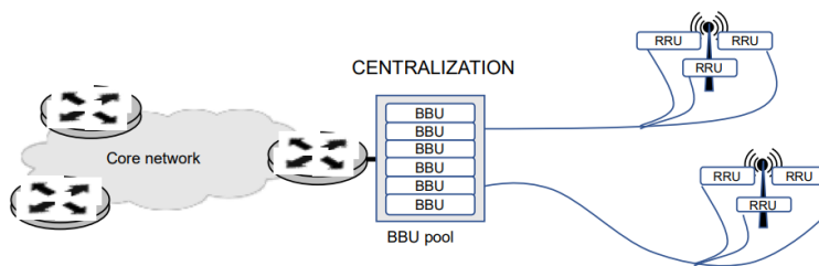
Х.1.2-р зураг - C-RAN ба уламжлалт бүтэц (“front-hauling” өмнөх)
