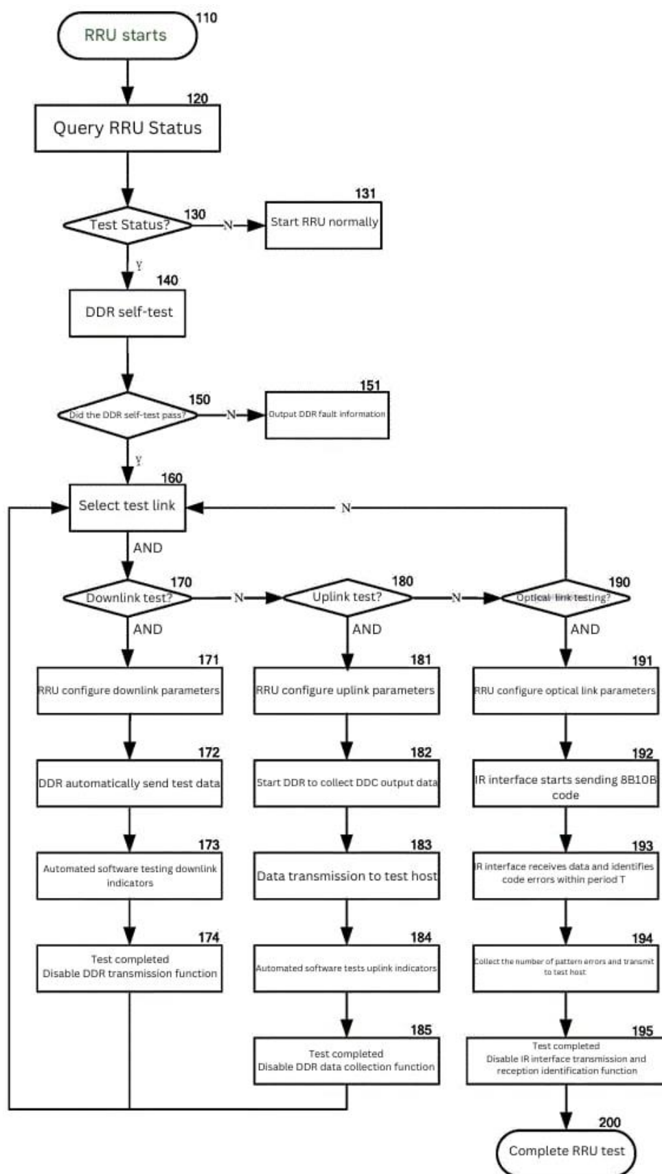
X.4.3-р зураг - RRU хэмжилтийн дэс дарааллын логик урсгал
