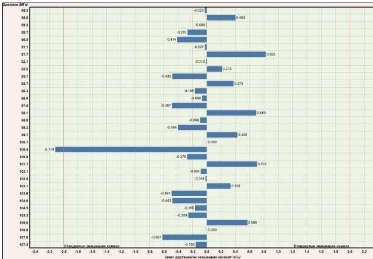
Зураг 7. Зөөгч давтамжийн зөвшөөрөх хазайлтын хэмжилтийн дүн.
