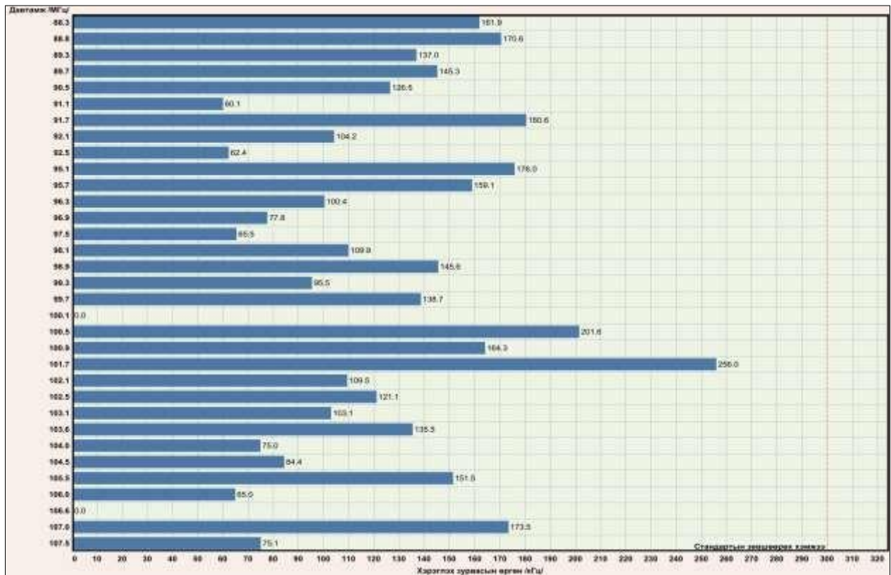
Зураг 5. Хэрэглэх зурвасын өргөний хэмжилтийн дүн.
