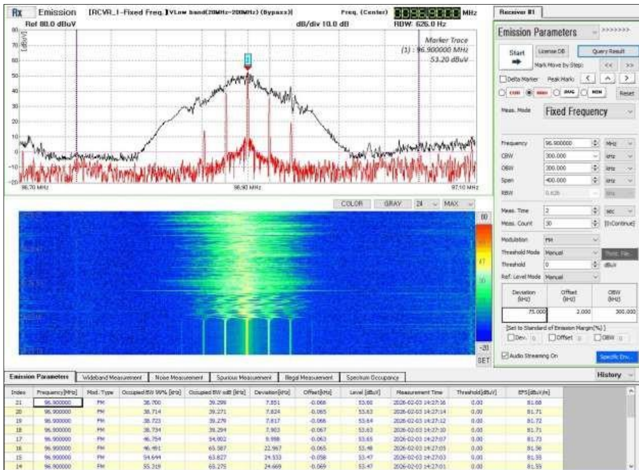
Зураг 4. FM радио станцын дохионы параметруудийн хэмжилт.
