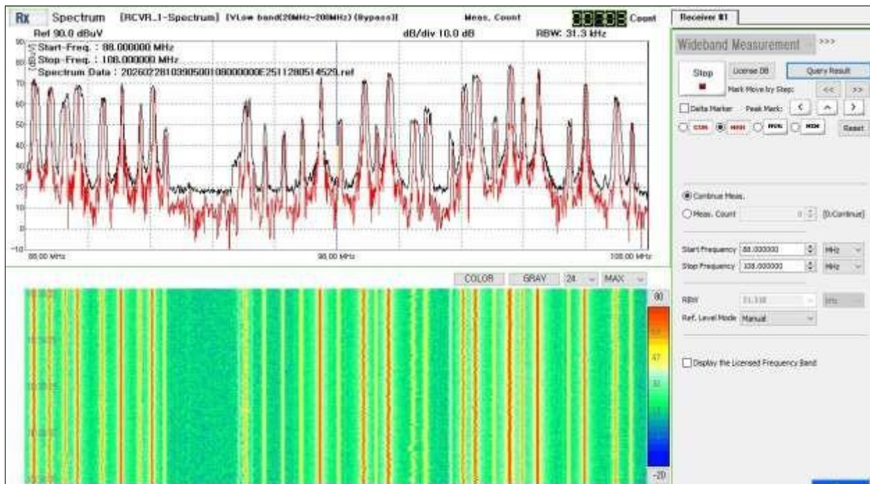
Зураг 3. Радио давтамжийн 88-108 МГц-ийн зурваст ажиллаж буй FM радио станцууд.
