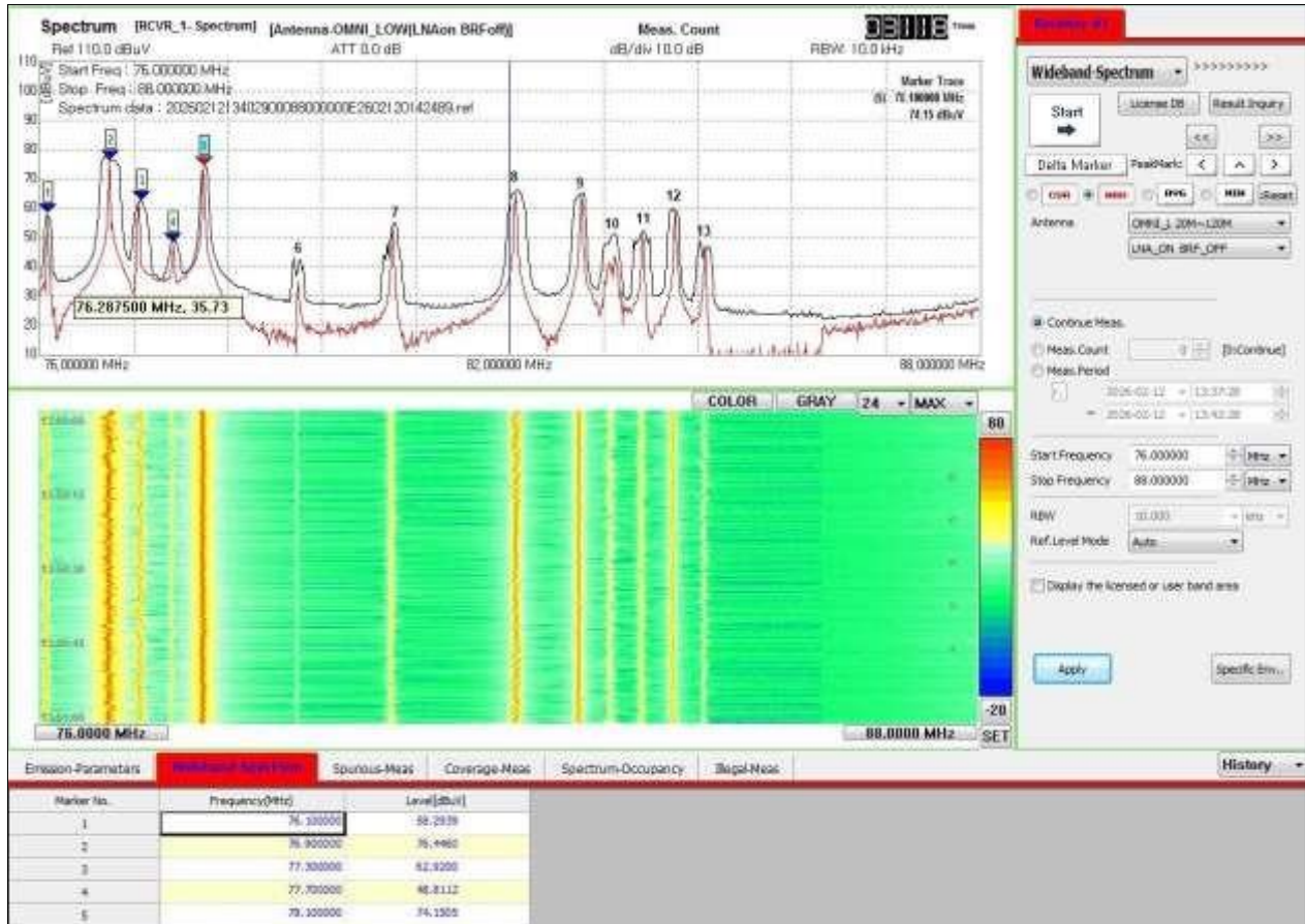
Зураг 8. Радио давтамжийн 76-87.5 МГц-ийн зурваст ажиллаж буй FM радиогийн дахин дамжуулах станцууд.
