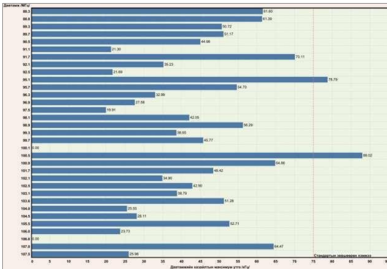
Зураг 6. Давтамжийн хазайлтын хэмжилтийн дүн.
