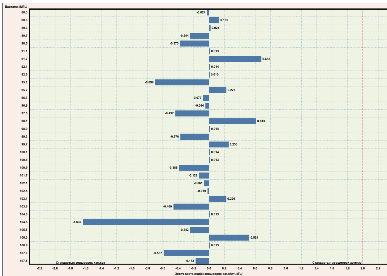
Зураг 4. Зөөгч давтамжийн зөвшөөрөх хазайлтын хэмжилтийн үр дүн
