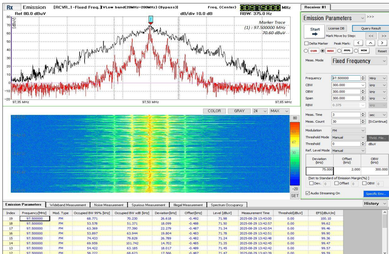
Зураг 3. Радио давтамжийн 88-108 МГц-ийн зурвасын хэмжилт
