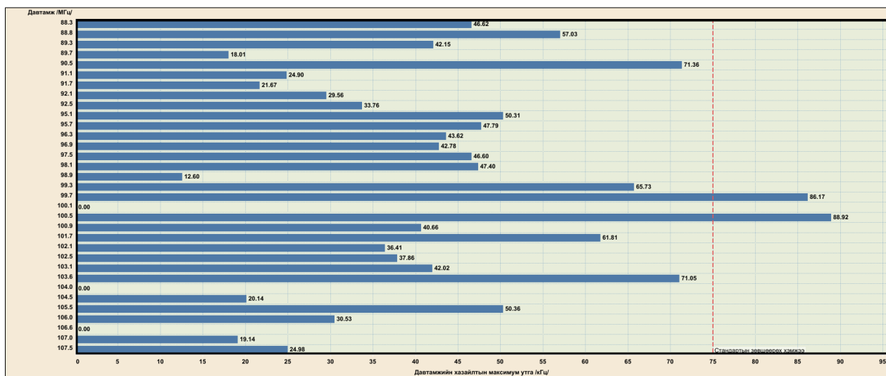
Зураг 6. Давтамжийн хазайлтын максимум утгын хэмжилтийн үр дүн
