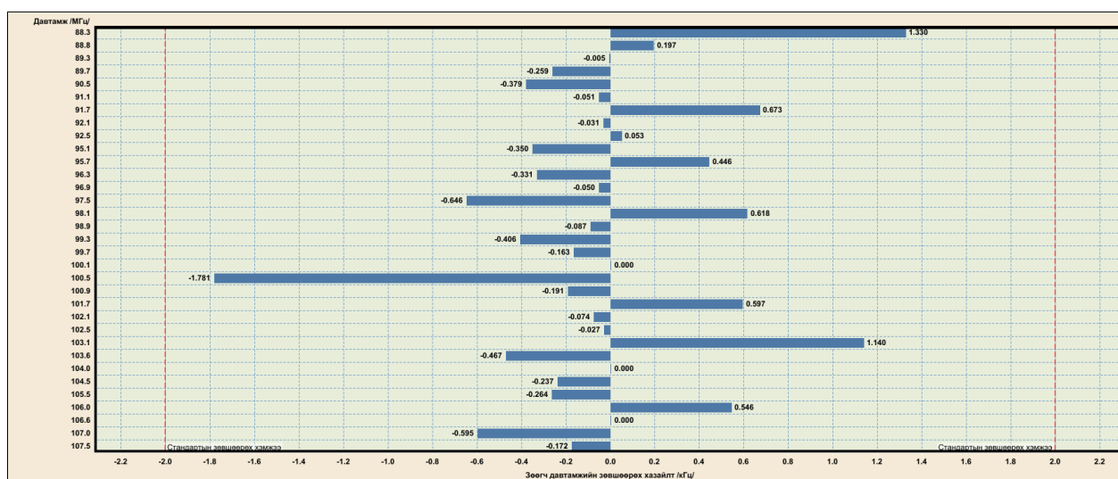
Зураг 4. Зөгч давтамжийн зөвшөөрөх хазайлтын хэмжилтийн үр дүн
