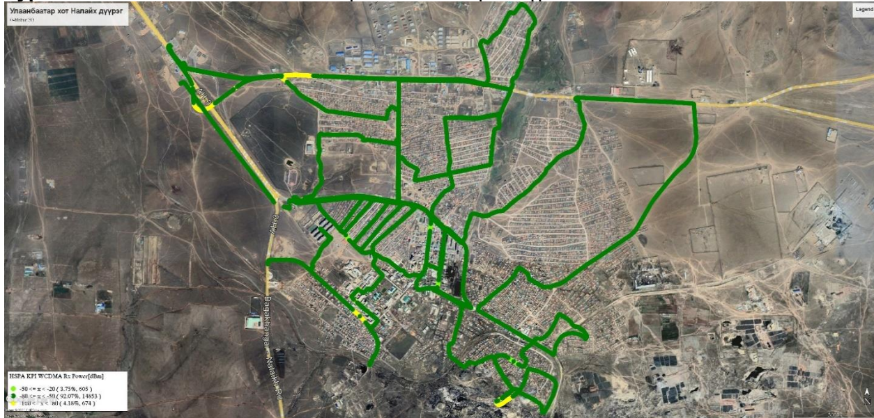
Зураг 2. “Жи-мобайл” ХХК-ийн 4G сүлжээний хамрах хүрээний хэмжилт
