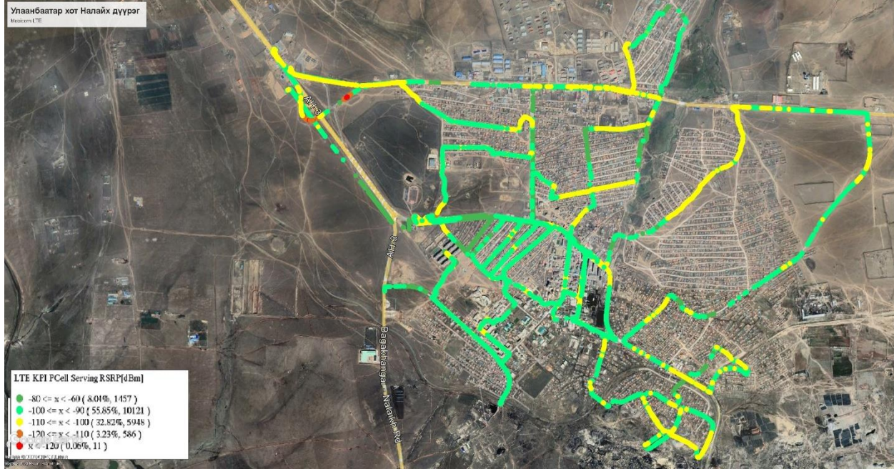
Зураг 3.1 Мобиком 4G хамрах хүрээний хэмжилт (LTE KPI RSRP[dBm])
