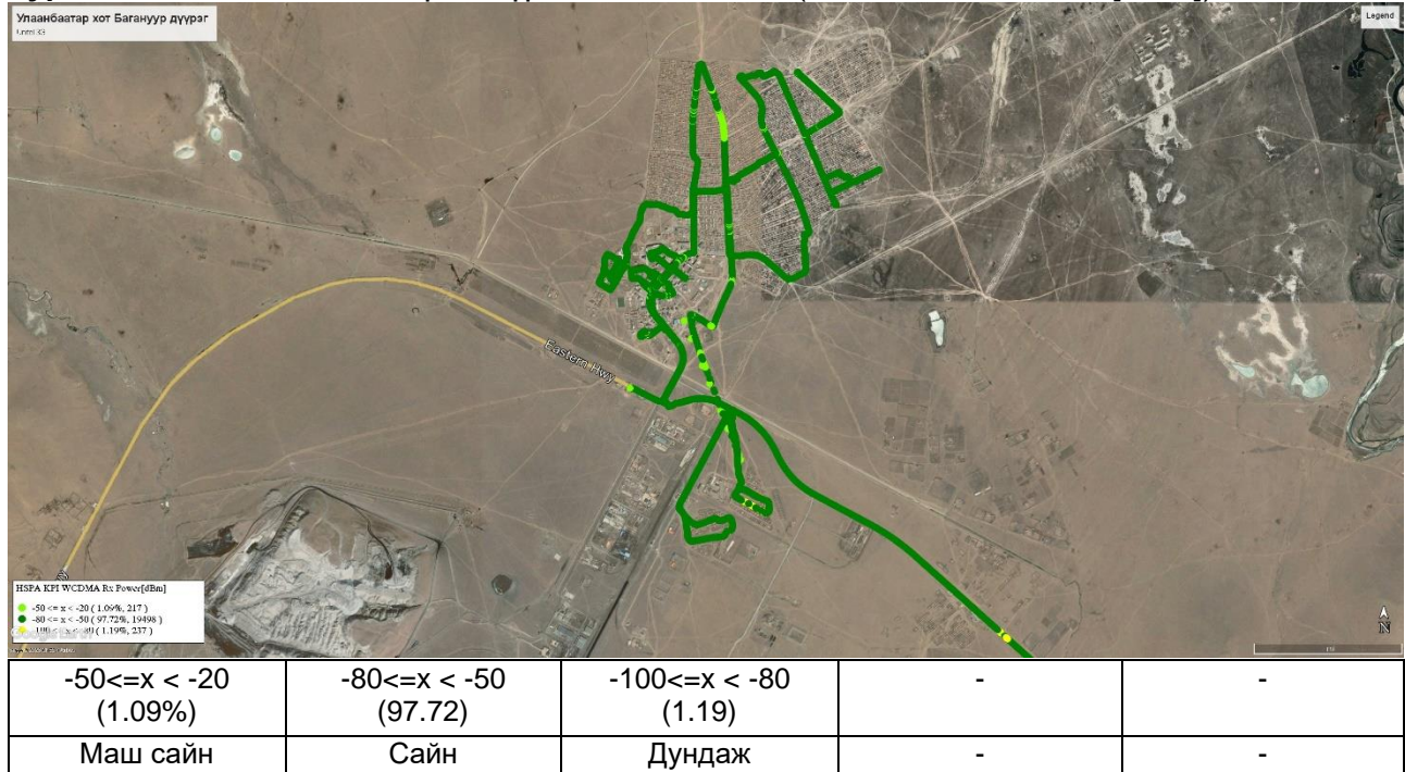
Зураг 3.2 Юнител 3G хамрах хүрээний хэмжилт (WCDMA Rx Power [dBm])
