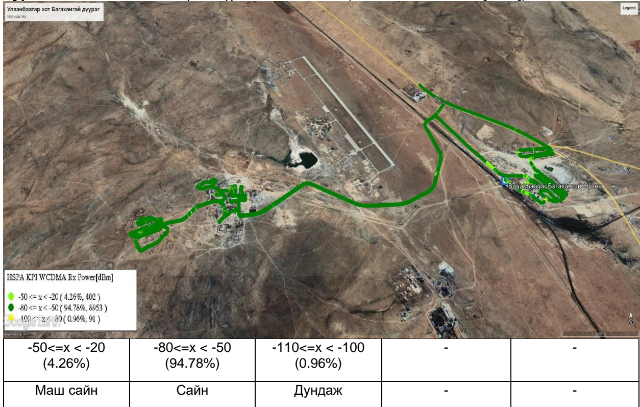
Зураг 2. Мобиком 3G хамрах хүрээний хэмжилт (WCDMA Rx Power [dBm])
