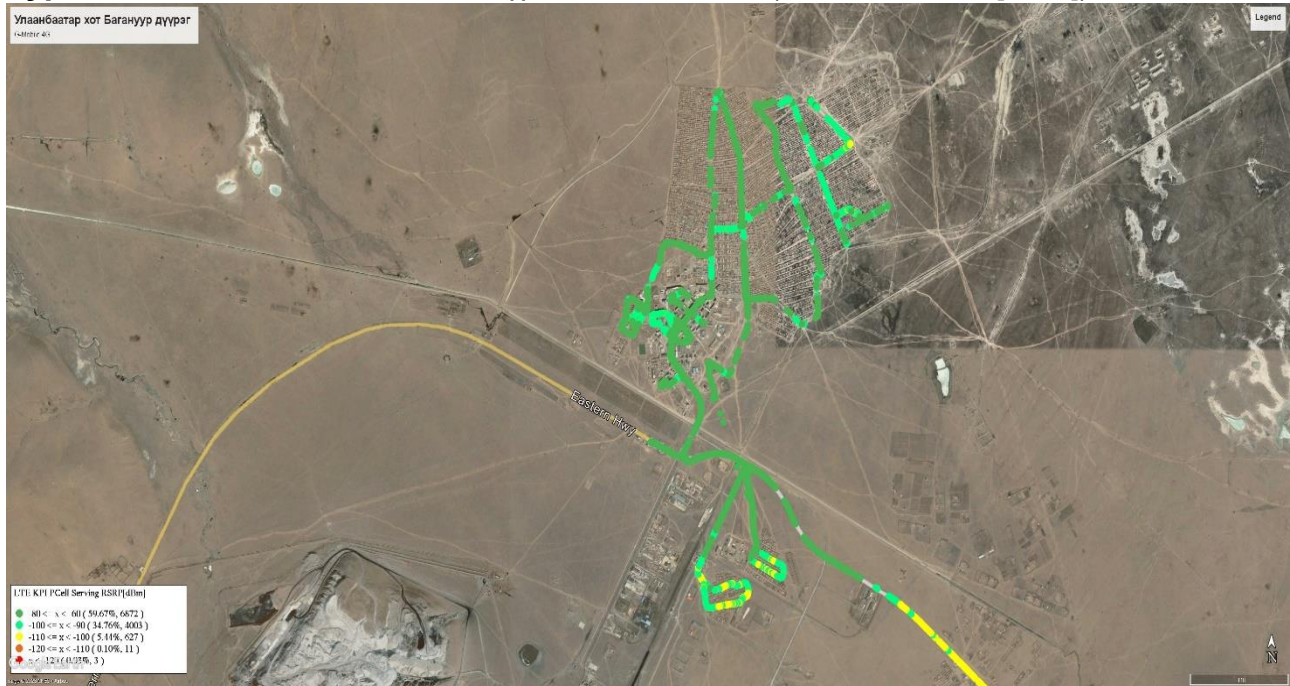
Зураг 2.1 Жи-Мобайл 4G хамрах хүрээний хэмжилт (LTE KPI RSRP[dBm])
