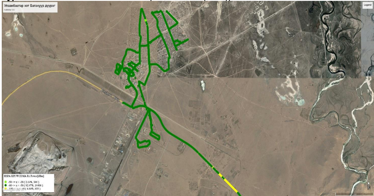
Зураг 2.2 “Жи-мобайл” ХХК-ийн 3G сүлжээний хамрах хүрээний хэмжилт
