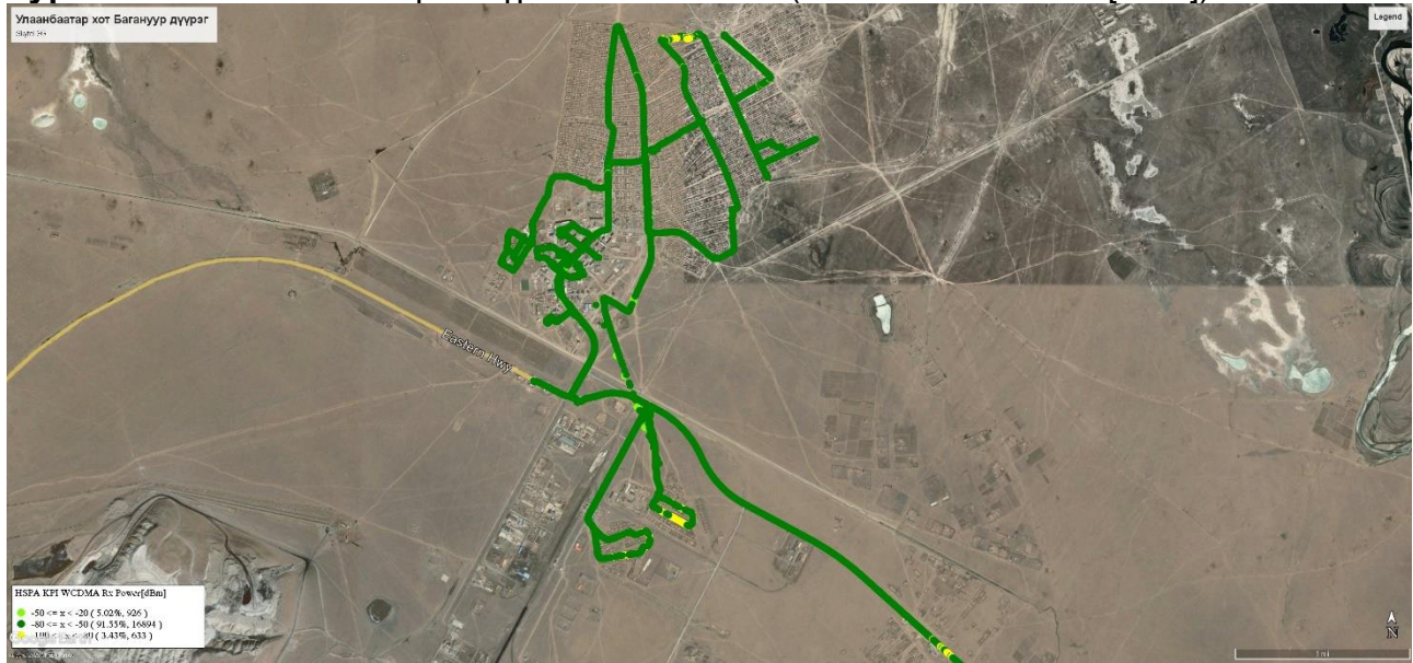
Зураг 2. Скайтел 3G хамрах хүрээний хэмжилт (WCDMA Rx Power [dBm])
