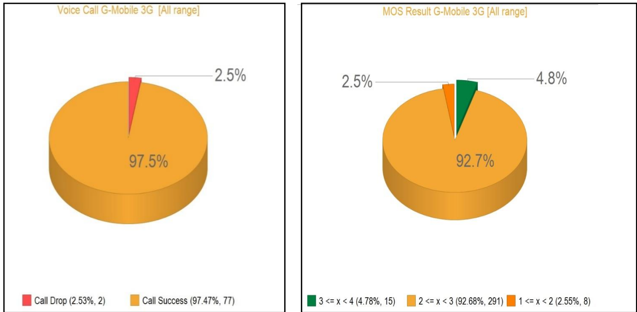
Зураг 3. “Жи-мобайл” ХХК-ийн 3G сүлжээний ярианы чанарын хэмжилт
