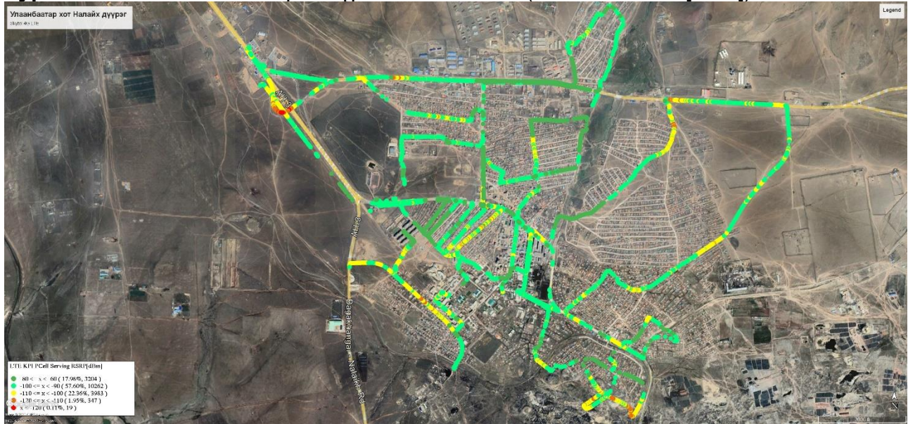
Зураг 3.1 Скайтел 4G хамрах хүрээний хэмжилт (LTE KPI RSRP[dBm])
