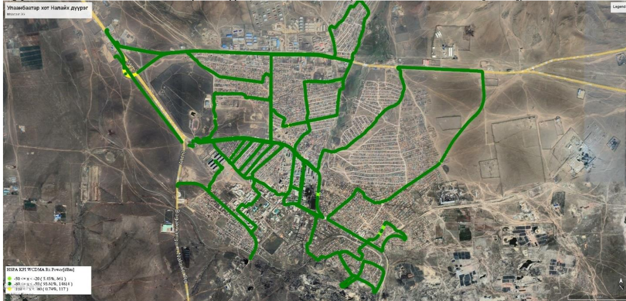
Зураг 3.2 Мобиком 3G хамрах хүрээний хэмжилт (WCDMA Rx Power [dBm])
