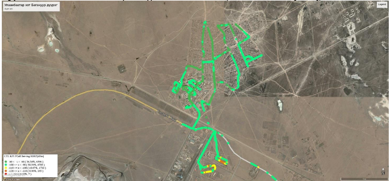
Зураг 2.1 Скайтел 4G хамрах хүрээний хэмжилт (LTE KPI RSRP[dBm])
