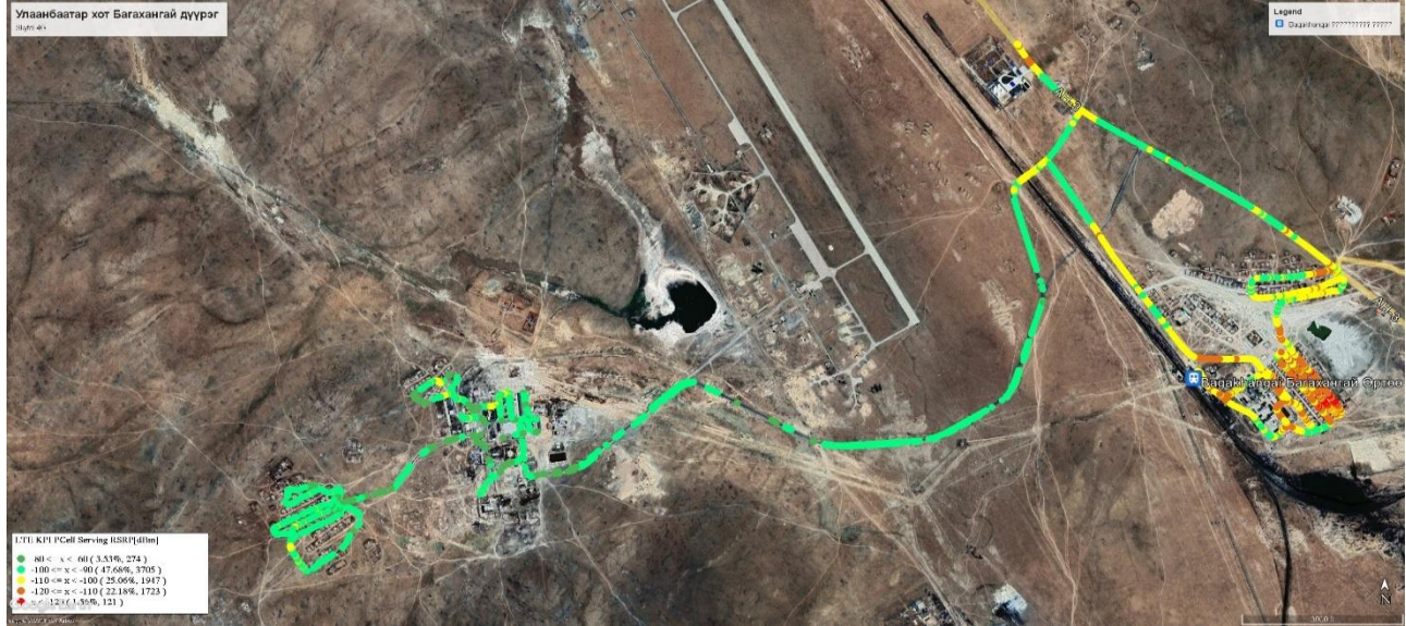
Зураг 1. Скайтел 4G хамрах хүрээний хэмжилт (LTE KPI RSRP[dBm])
