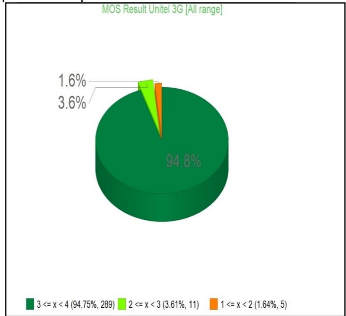
Зураг 2.3 “Юнител” ХХК-ийн 3G сүлжээний ярианы чанарын хэмжилт
