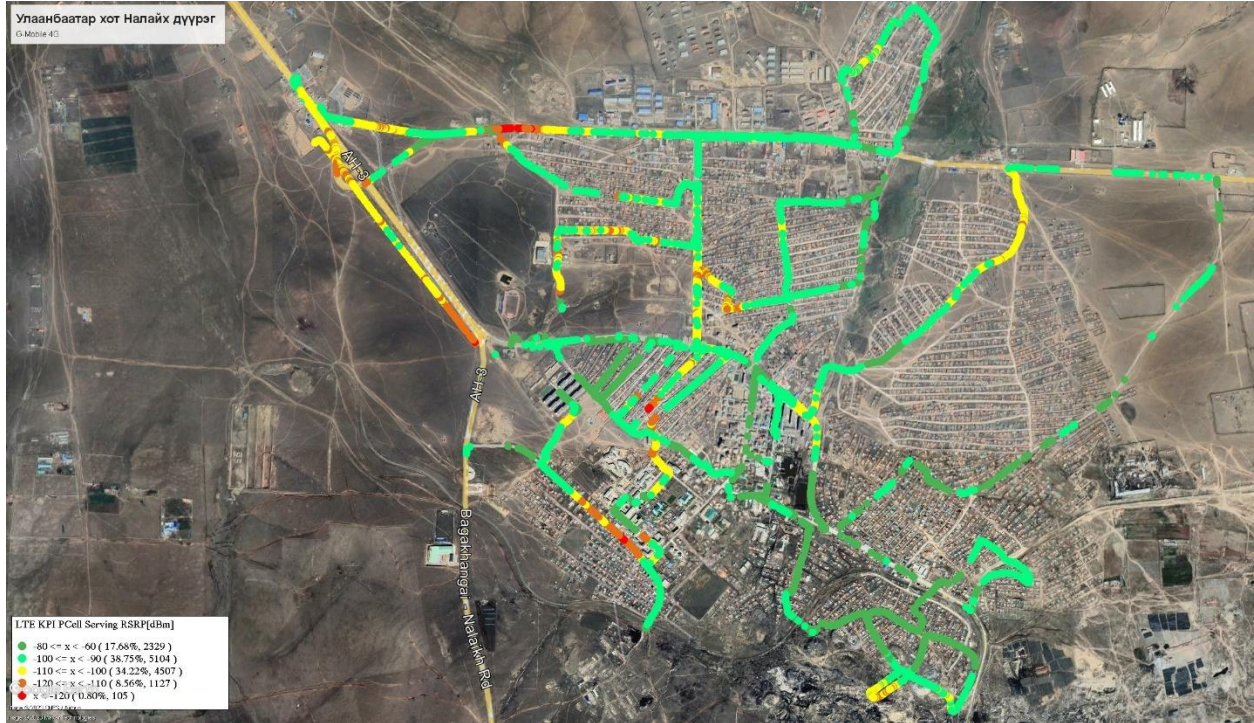
Зураг 1. Жи-Мобайл 4G хамрах хүрээний хэмжилт (LTE KPI RSRP[dBm])
