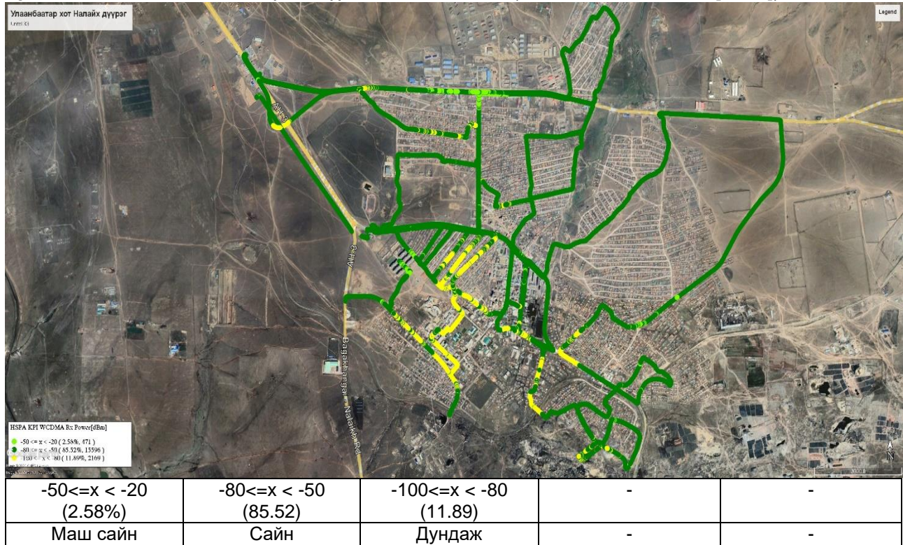
Зураг 2.2 Юнител 3G хамрах хүрээний хэмжилт (WCDMA Rx Power [dBm])
