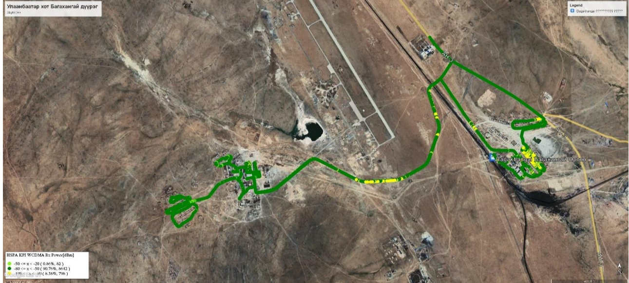
Зураг 2. Скайтел 3G хамрах хүрээний хэмжилт (WCDMA Rx Power [dBm])
