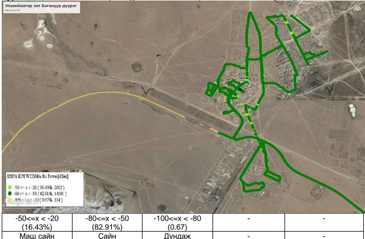
Зураг 2.2 Мобиком 3G хамрах хүрээний хэмжилт (WCDMA Rx Power [dBm])
