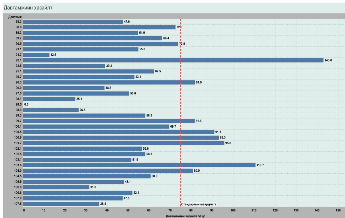
Зураг 3. Давтамжийн модуляцтай дохионы давтамжийн хазайлтын утга
