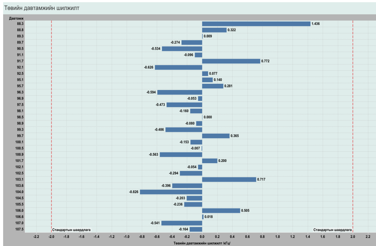
Зураг 4. Нэвтрүүлэгчийн зөөгч давтамжийн зөвшөөрөх хазайлт
