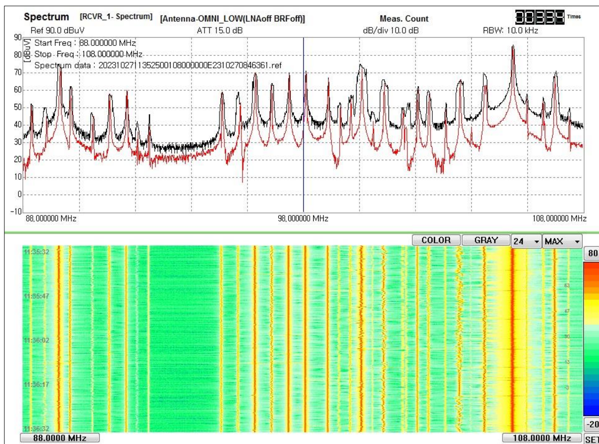
Зураг 2. Хэмжилт хийх үеийн зураг.
