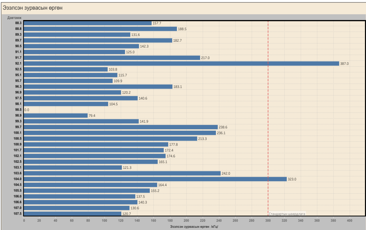
Зураг 5. Эзэлсэн зурвасын өргөн
