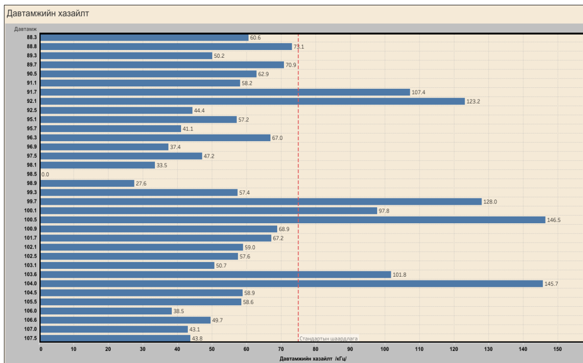
Зураг 3. Давтамжийн модуляцтай дохионы давтамжийн хазайлтын утга
