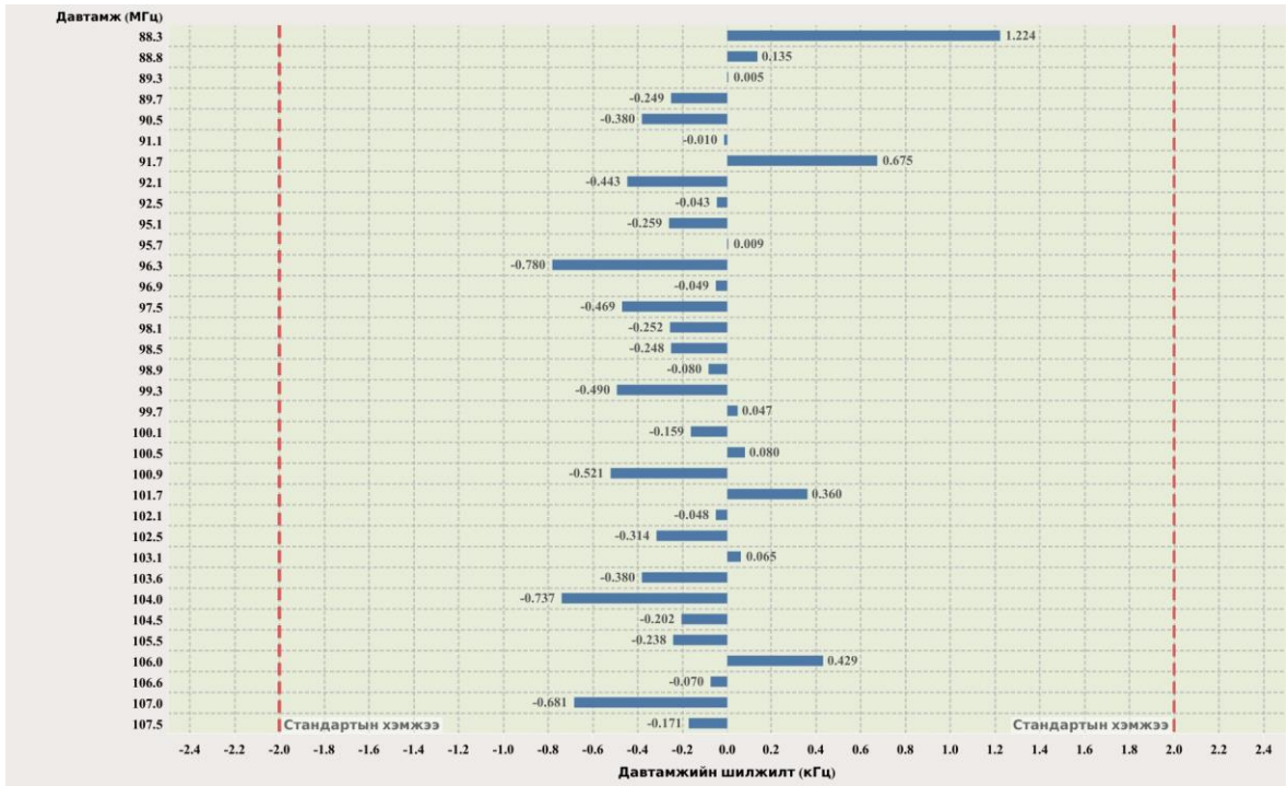
Зураг 4. Нэвтрүүлэгчийн зөөг давтамжийн зөвшөөрөх хазайлт.
