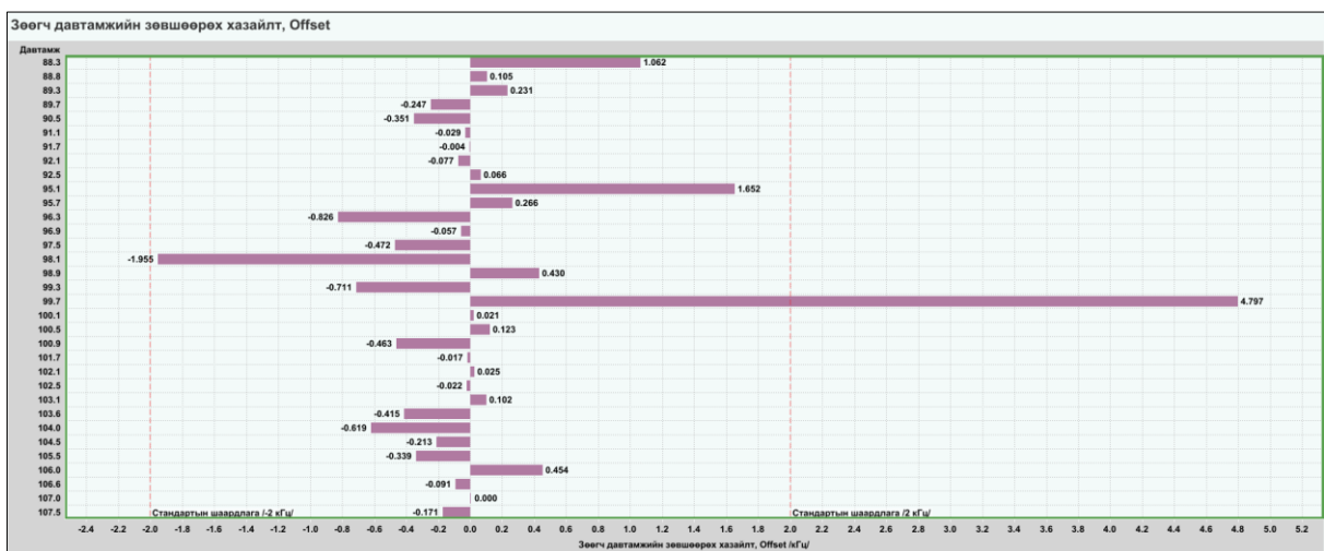
Зураг 5. Зөөгч давтамжийн зөвшөөрөх хазайлтын хэмжилтийн үр дүн
