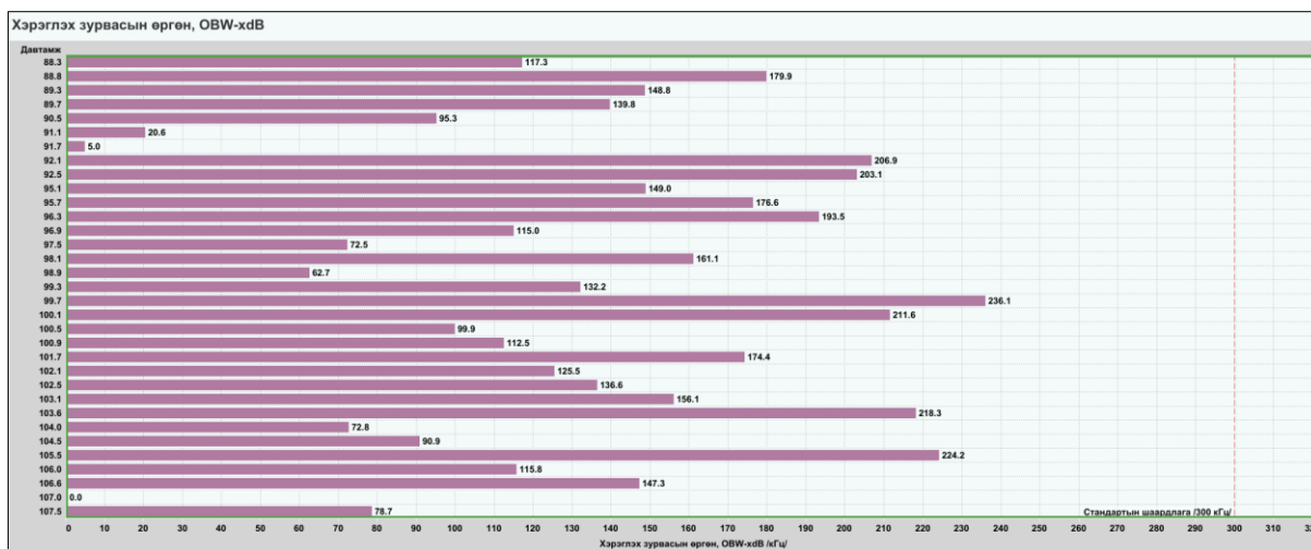
Зураг 6. Хэрэглэх зурвасын өргөний хэмжилтийн үр дүн
