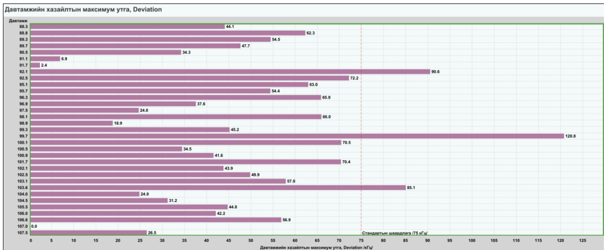
Зураг 4. Давтамжийн хазайлтын максимум утгын хэмжилтийн үр дүн
