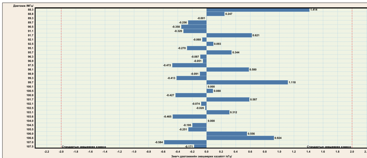
Зураг 4. Зөөгч давтамжийн зөвшөөрөх хазайлтын хэмжилтийн үр дүн
