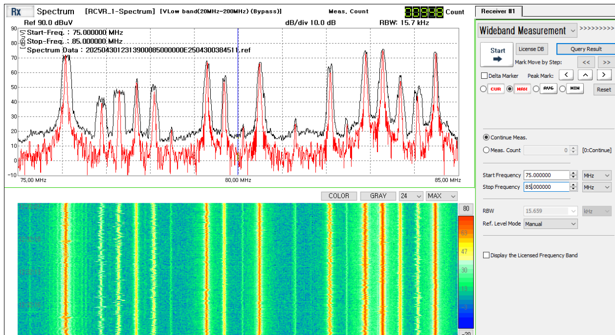
Зураг 7. Радио давтамжийн 75 МГц-85 МГц-ийн зурвасын хэмжилт
