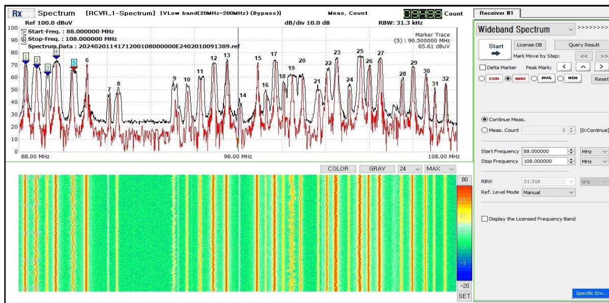
Зураг 2. Радио давтамжийн 88 МГц-108.0 МГц-ийн зурвасын хэмжилт
