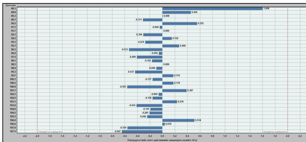
Зураг 3. Зөөгч давтамжийн зөвшөөрөх хазайлтын хэмжилтийн үр дүн
