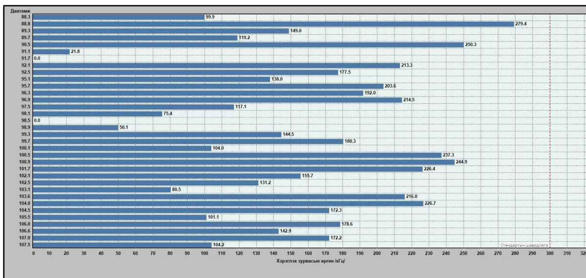
Зураг 4. Хэрэглэх зурвасын өргөний хэмжилтийн үр дүн
