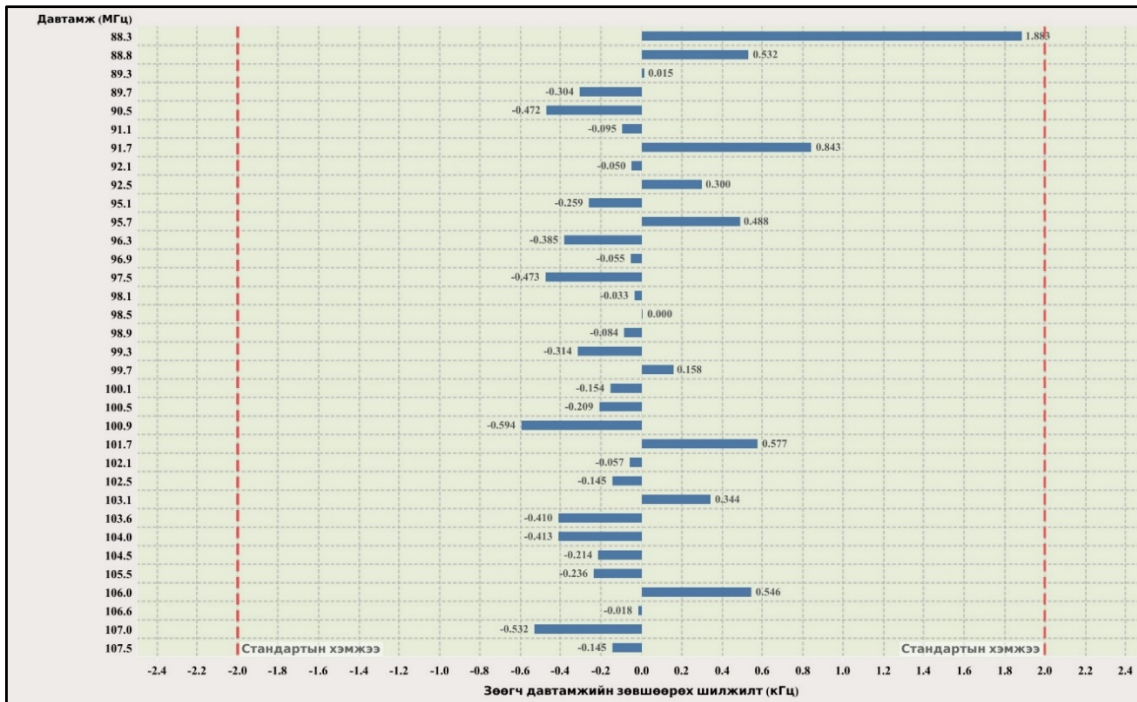
Зураг 4. Зөөгч давтамжийн зөвшөөрөх хазайлт нь стандартын шаардлагыг хангасан FM радио нэвтрүүлэх станцууд.
