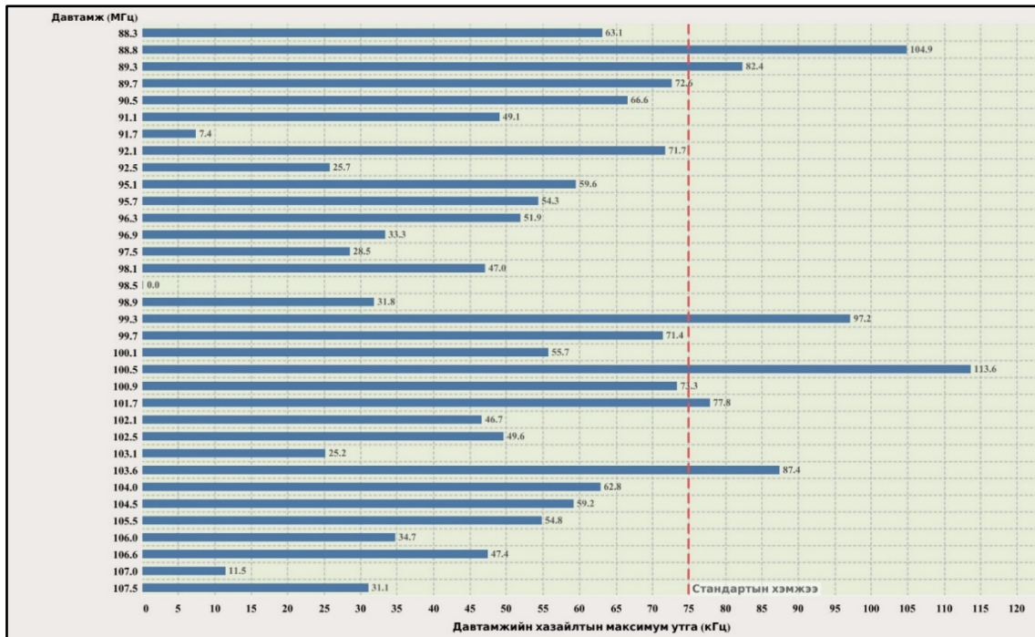
Зураг 5. Давтамжийн хазайлтын максимум утга нь стандарт хэмжээнээс хэтэрсэн FM радио нэвтрүүлэх станцууд.
