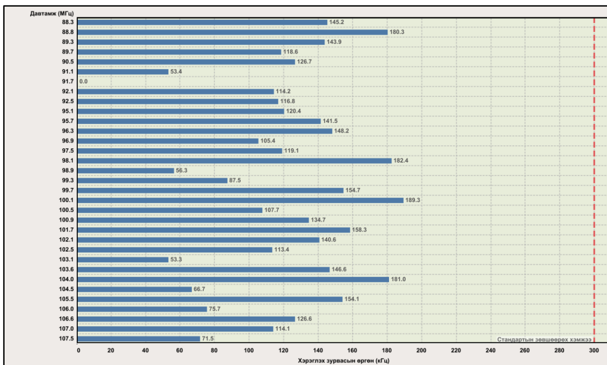
Зураг 5. Хэрэглэх зурвасын өргөний хэмжилтийн үр дүн
