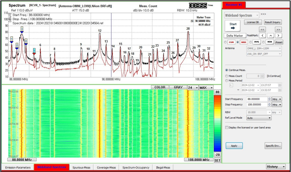
Зураг 2. Радио давтамжийн 88 МГц-108.0 МГц-ийн зурвасын хэмжилт
