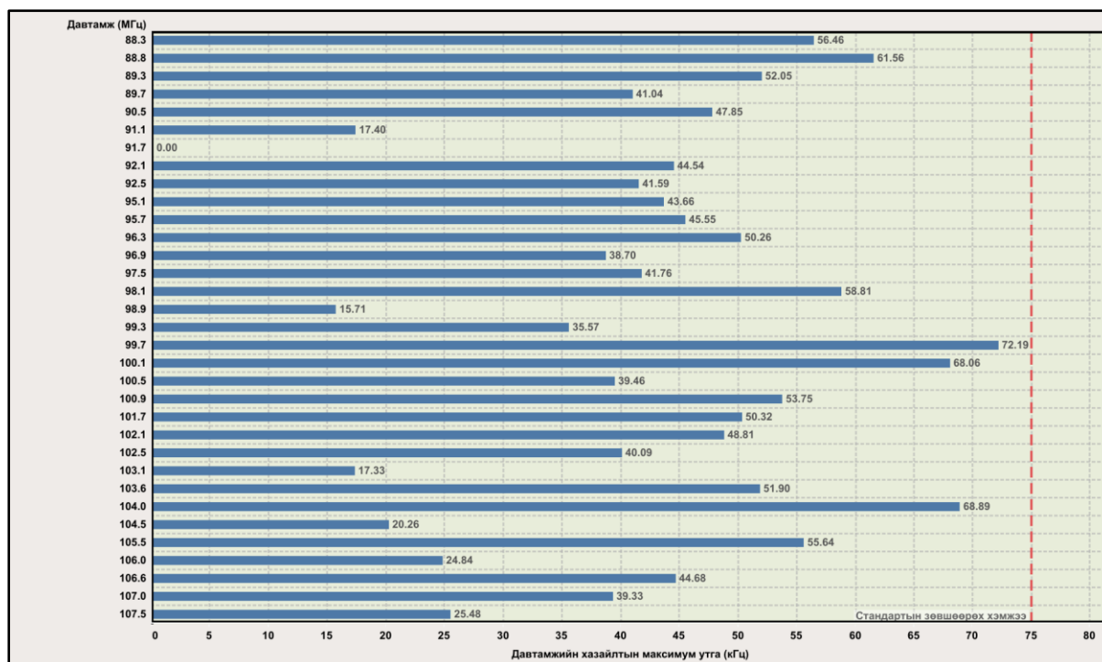
Зураг 3. Давтамжийн хазайлтын максимум утгын хэмжилтийн үр дүн
