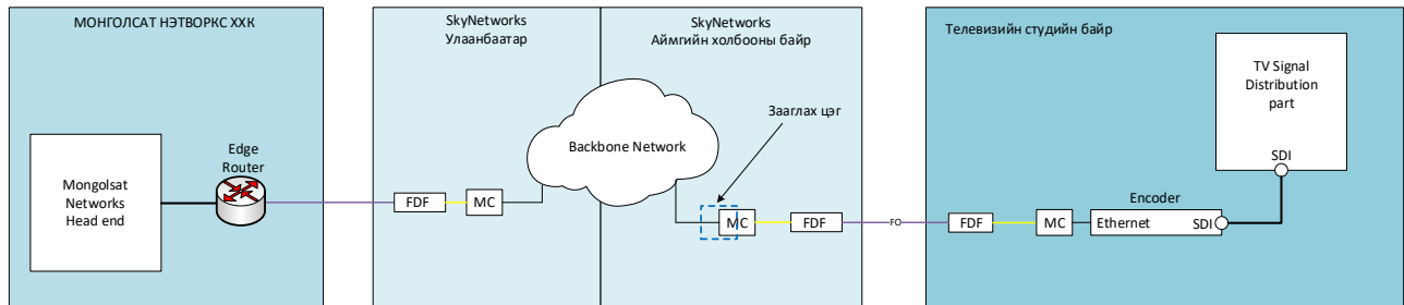
4.3 Орон нутгийн телевизийн холболт хийх зураглал (Байршил 3)
