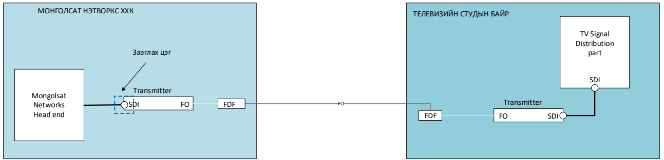
4.3 Орон нутгийн телевизийн холболт хийх зураглал (Байршил 3)
